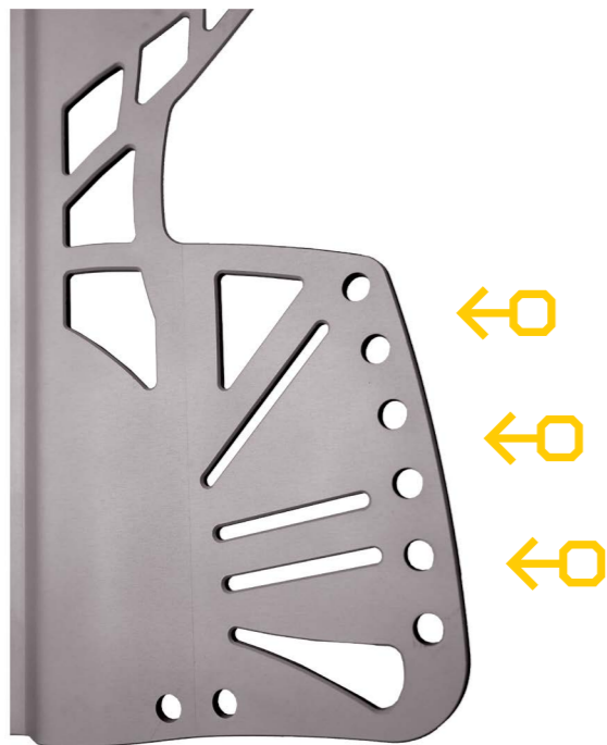
Rys.4. Punkty mocowania kieszeni balastowych
