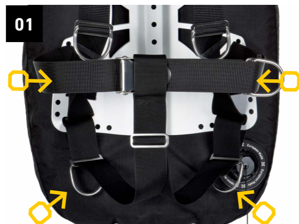
Rys. 8. Miejsca regulacji pasów naramiennych i pasa kroczyzny w standardowej uprzęży.
